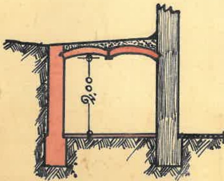
Schnitt a-b.
